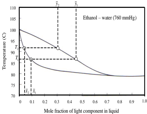
รูปที่ 1 แผนภาพสมดุลของของผสมไอ - ของเหลวที่มี 2 องค์ประกอบ ภายใต้สภาวะความดันคงที่
